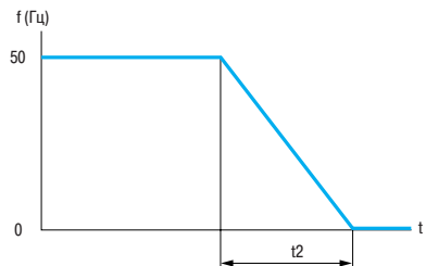
Линейная кривая торможения
